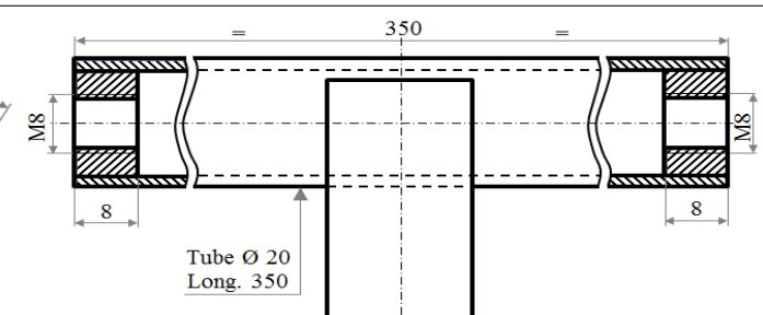
Vue de gauche (Support avant)
